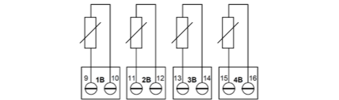
i | Collegamento come 4 ingressi configurabili singolarmente per sonde di temperatura passive (NTC 10 kΩ a 25 °C).
