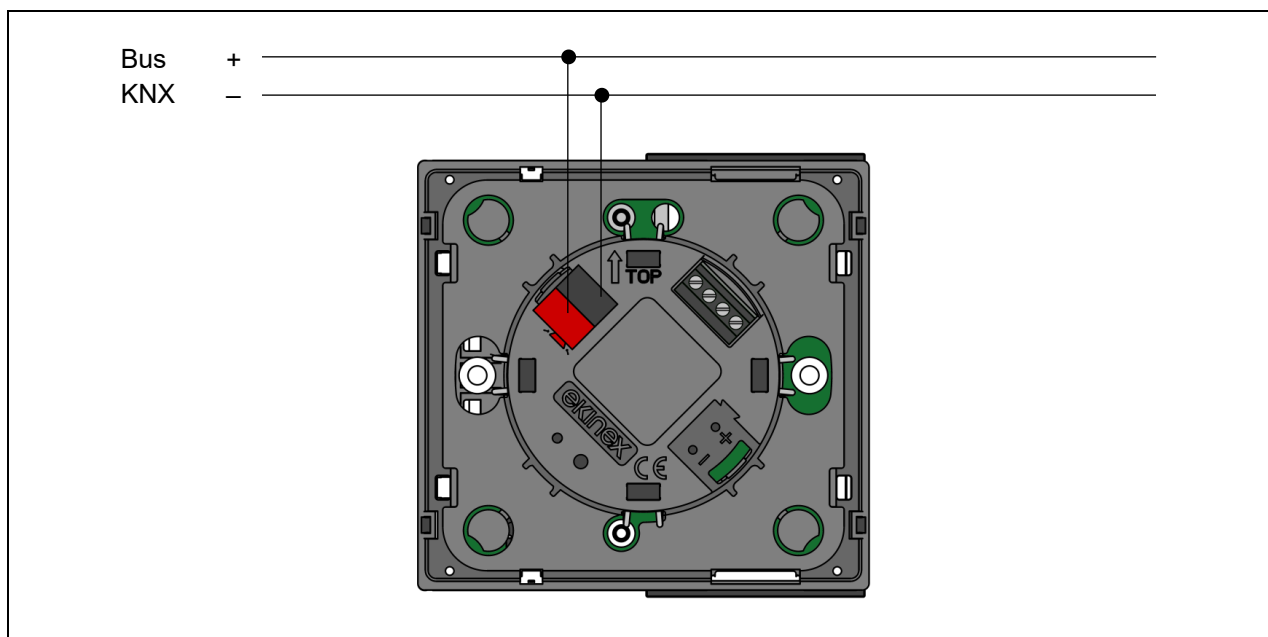
Collegamento dell'apparecchio alla linea bus
