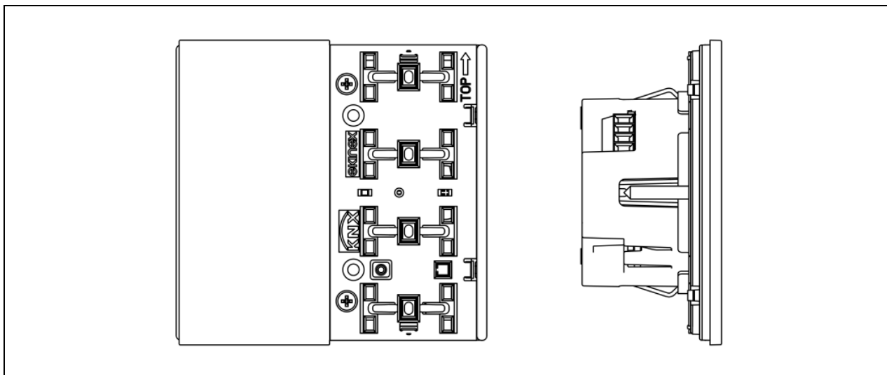
Esecuzione dell'apparecchio: vista frontale e laterale
