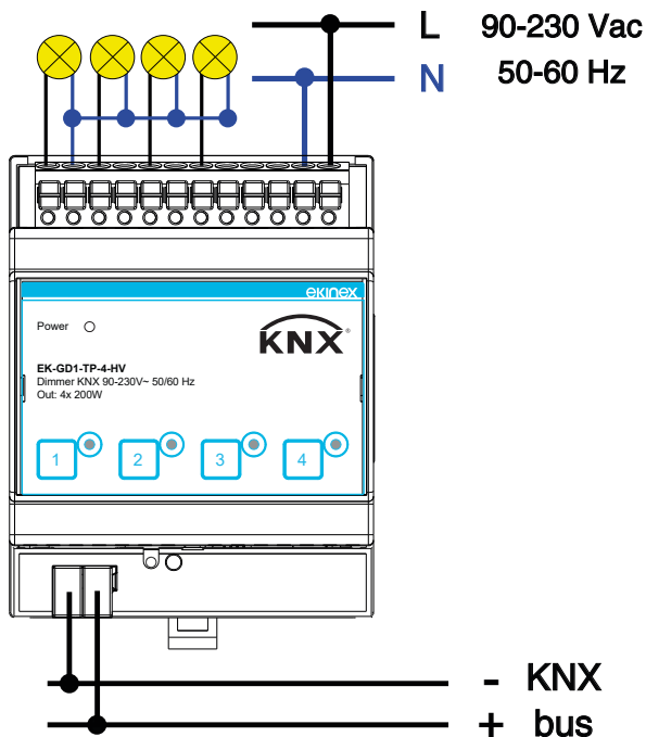
Schema di installazione con uscite a collegamento del polo COM in comune
